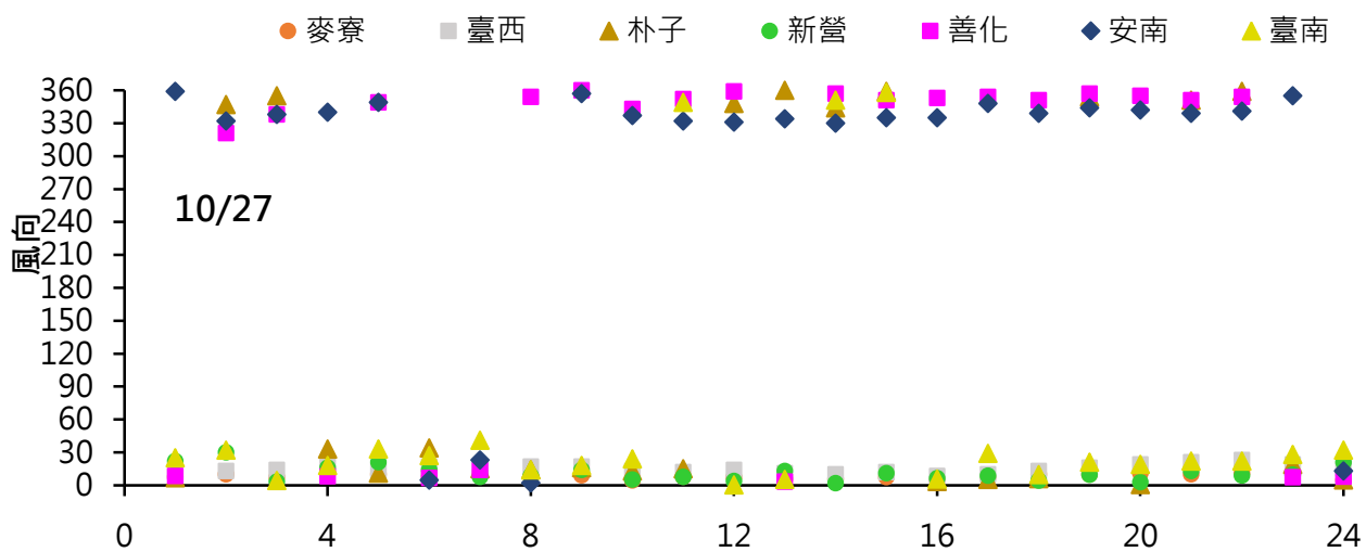
圖 7、107/2/27~3/1 本市測站 PM 2.5 濃度、風速及風速逐時變化
