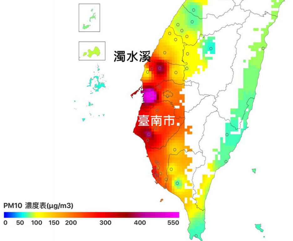
圖 7、107 年 10 月 27 日 14 時-19 時 PM 10 濃度平均潛勢圖
