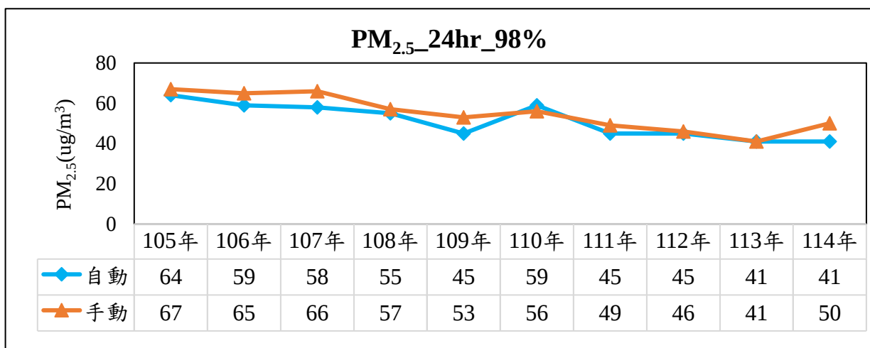
圖5、本市嘉義測站105-114年 PM 2.5 24小時值(Pr98)變化趨勢
