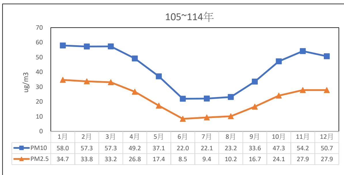
圖6、本市嘉義測站105-114年 PM 10 及 PM 2.5 月濃度平均變動趨勢
