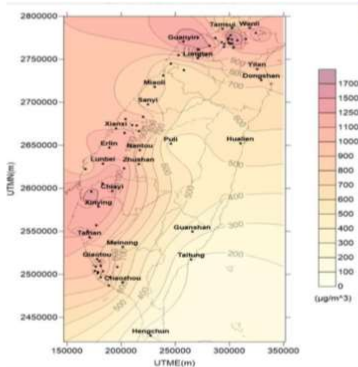
圖 13、99 年 3 月 21 日大陸沙塵暴事件 PM 10 小時最大濃度分布
