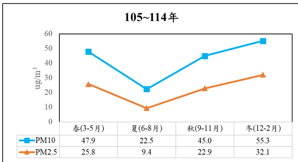
圖7、本市嘉義測站105-114年 PM 10 及 PM 2.5 季節變動趨勢
