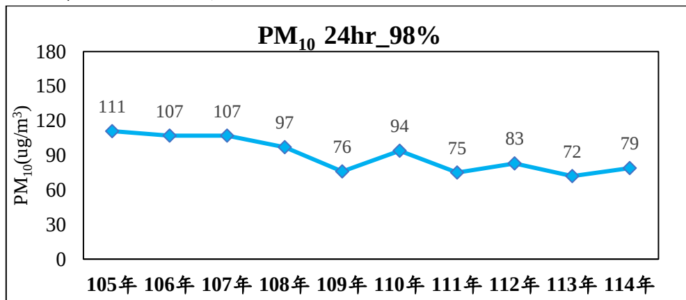
圖4、本市嘉義測站105-114年 PM 10 24小時值(Pr98)變化趨勢
